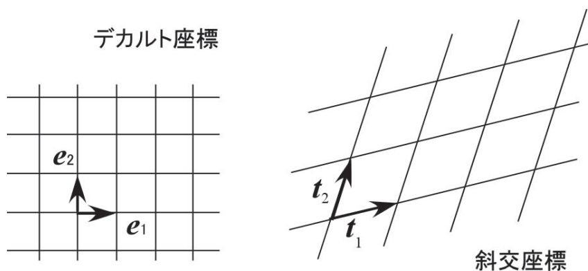
図 1.5: 斜交座標系
