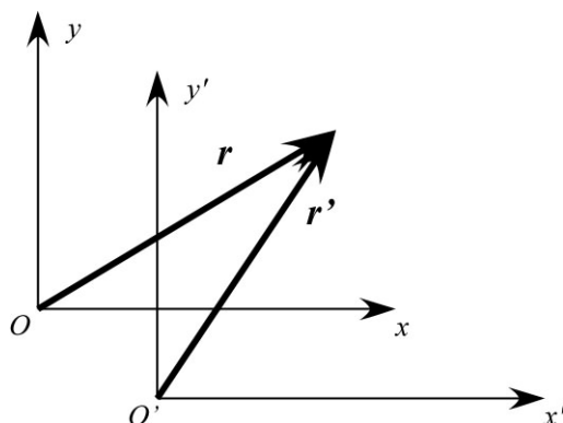
図 1.15: 平行移動による位置ベクトルの変化
