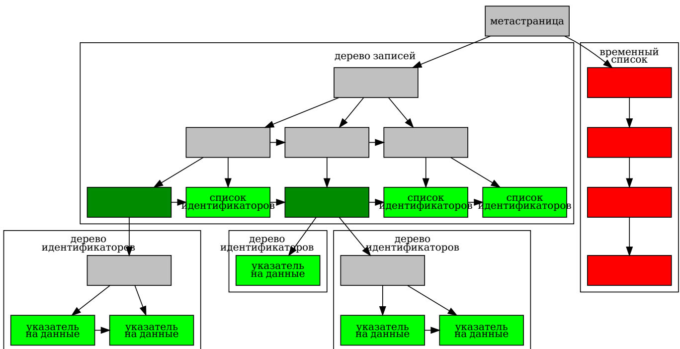
Рисунок 64.1. Внутреннее устройство GIN
