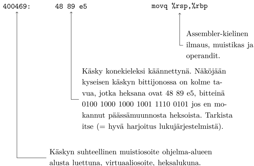
Kuva 11: Assembler-rivin rakenne, jossa näky osoite, konekielinen tavuesitys ja assembler-käskey GNU Assemblerin mukaisena.
