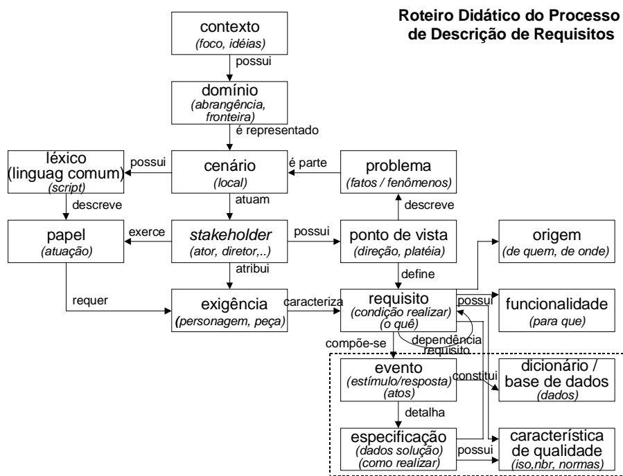
Figura 2 - Roteiro Didático do Processo de Descrição de Requisitos
