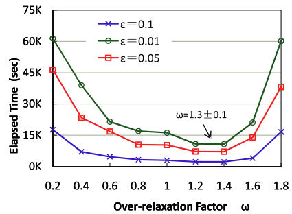
(d) Relaxation Factor ( n = 10K )
