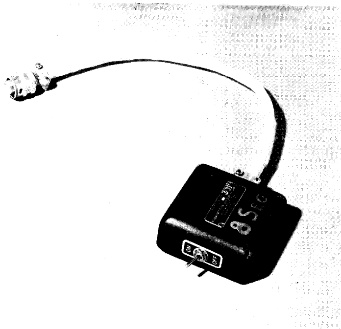
Figure 4.14-2 - 8-Second Intervalometer (-302)
