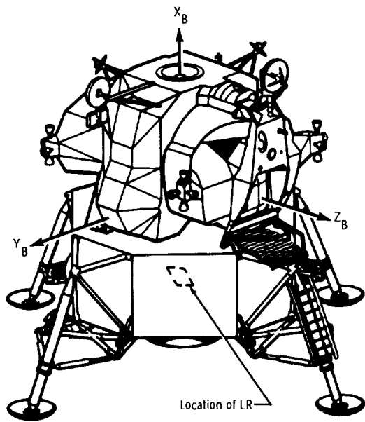
(a) Lunar module body axes.
