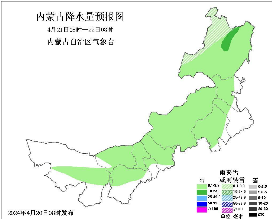
图4 2024年4月21日08时-4月22日08时内蒙古降水量预报图
