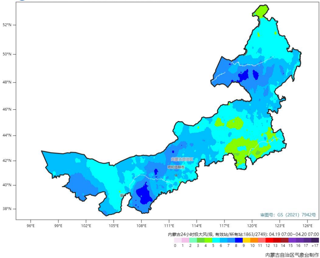
图 2 2024 年 4 月 19 日 07 时-4 月 20 日 07 时内蒙古大风实况图
