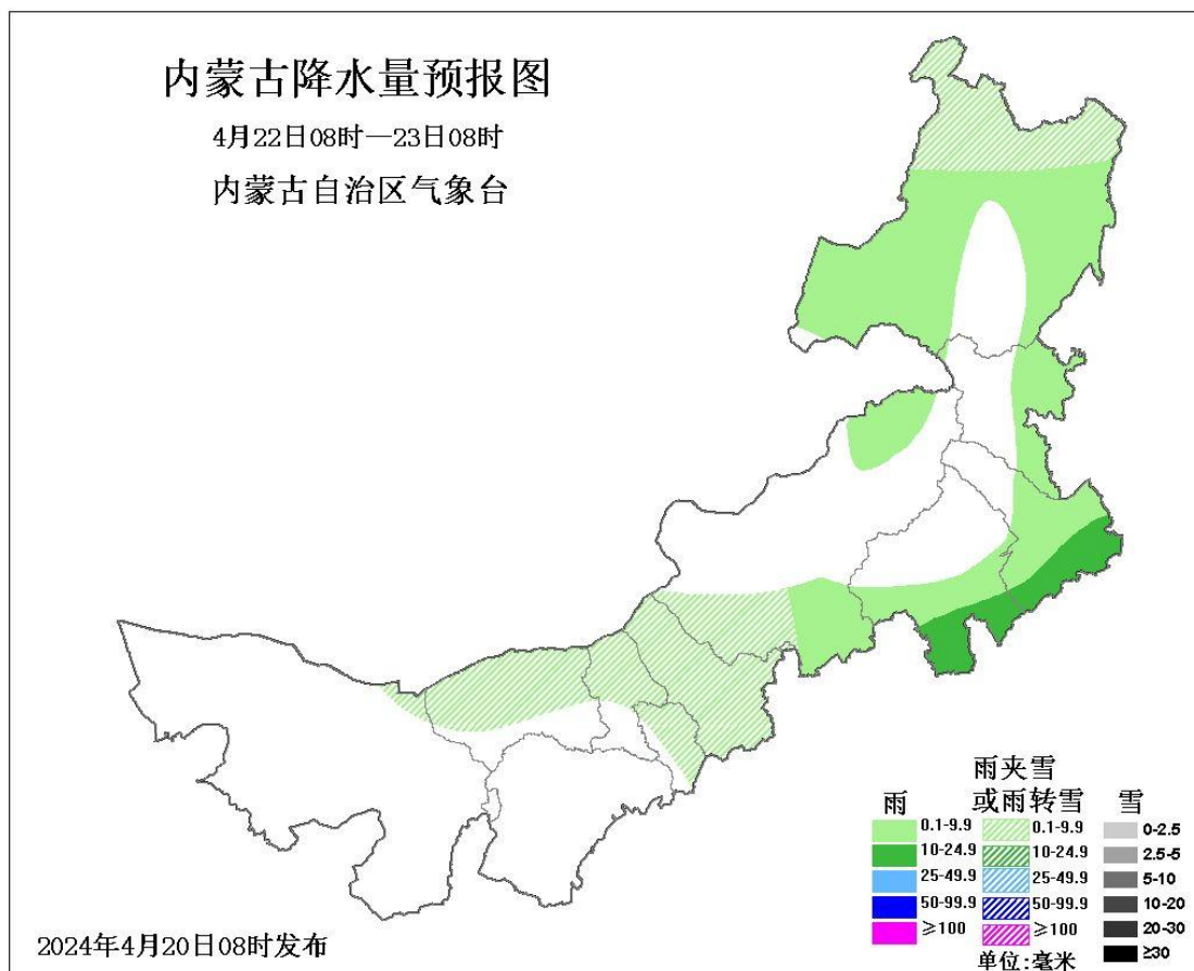
图5 2024年4月22日08时-4月23日08时内蒙古降水量预报图
