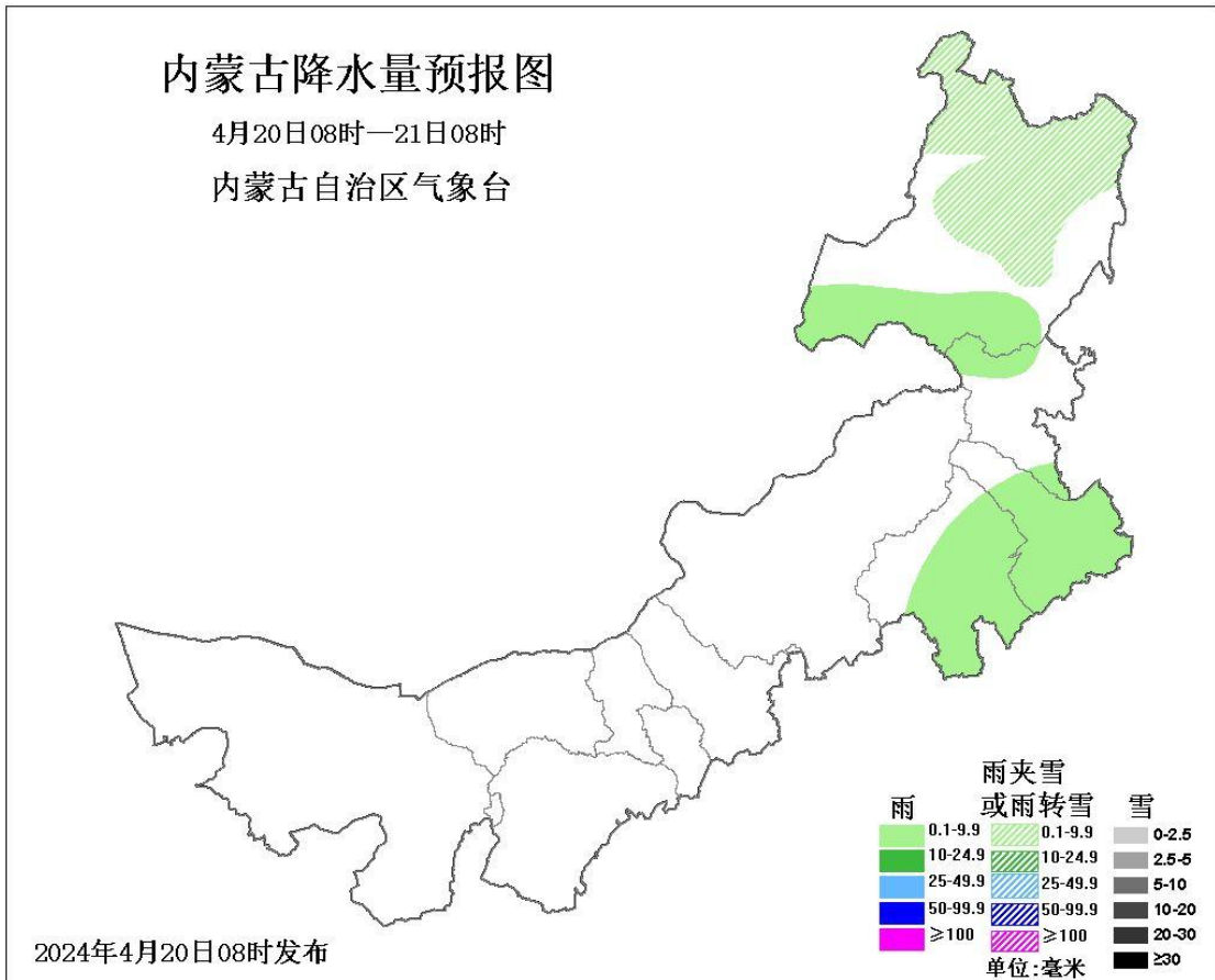
图3 2024年4月20日08时-4月21日08时内蒙古降水量预报图
