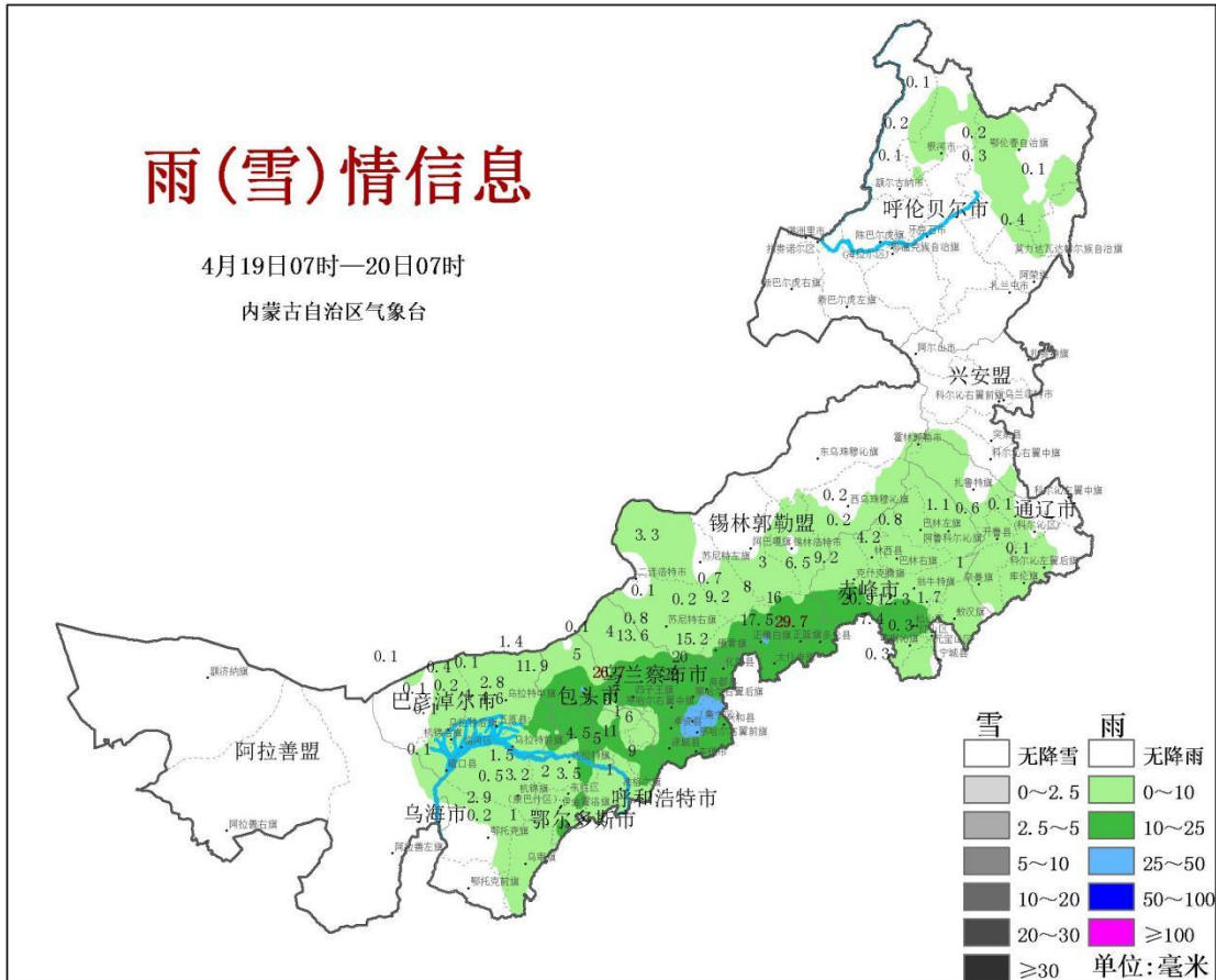
图1 2024年4月19日07时-4月20日07时内蒙古降水实况图
