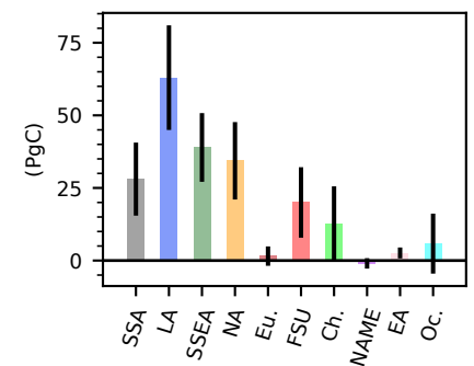
Cum. ELUC (1750-2018)
