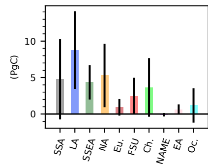
Cum. LASC (1750-2018)
