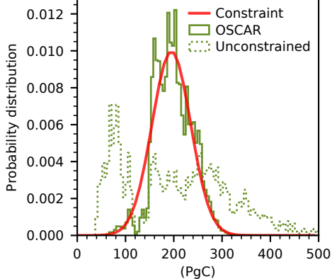
(d) Cum. LULCC emissions (1850–2018)
