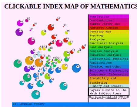
Fig. 1: Rusin’s Math Atlas [Rus01]
