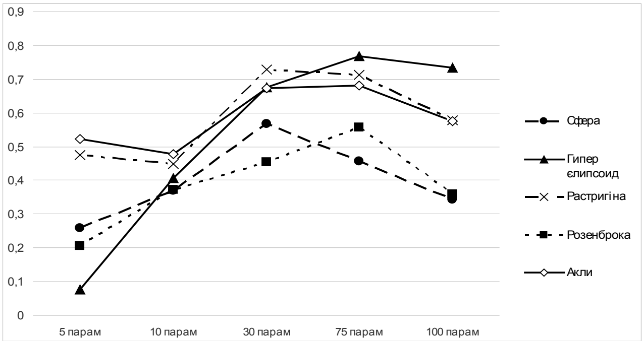
Рис. 5. S-оцінка часової ефективності алгоритмів зі зростанням кількості епох
