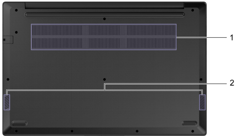
Figure 15. Bottom view—Lenovo V15 G4 IRU, Lenovo V15 G4 IAH, Lenovo V15 G4 IRH and Lenovo V15 G4 ABP
