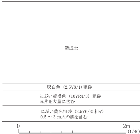
図 20 A地点土層断面柱状図
