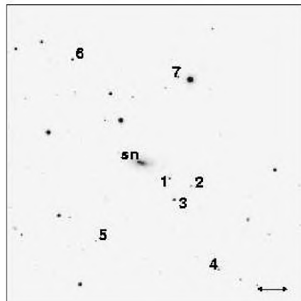
SN 1998dk
