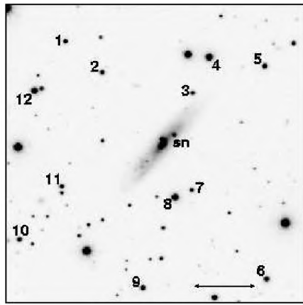
SN 1999gp
