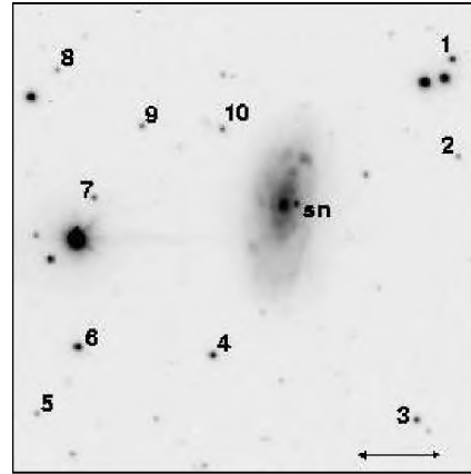
SN 1997dt
