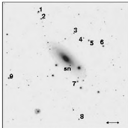
SN 1998D
