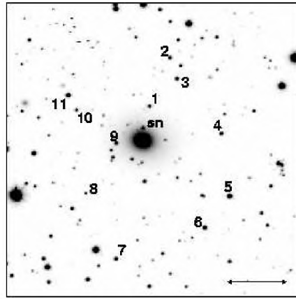
SN 1998bp
