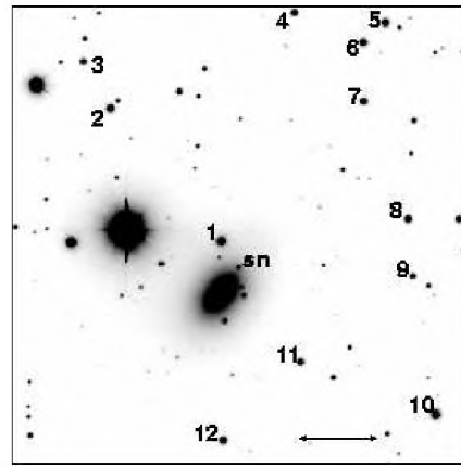
SN 2000B
