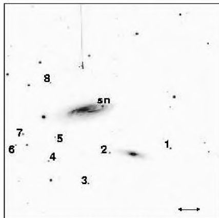
SN 1998dh
