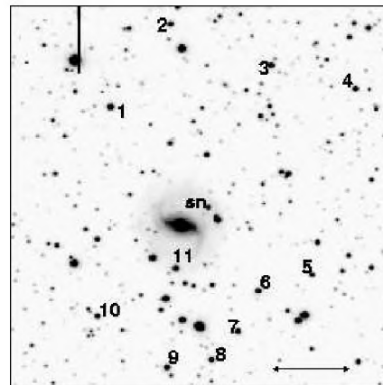
SN 1998V
