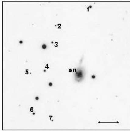
SN 1997cw
