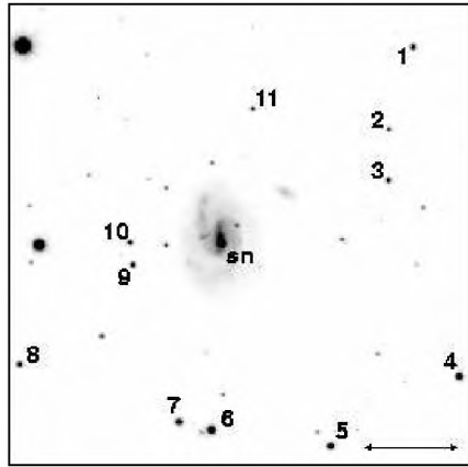
SN 1997do
