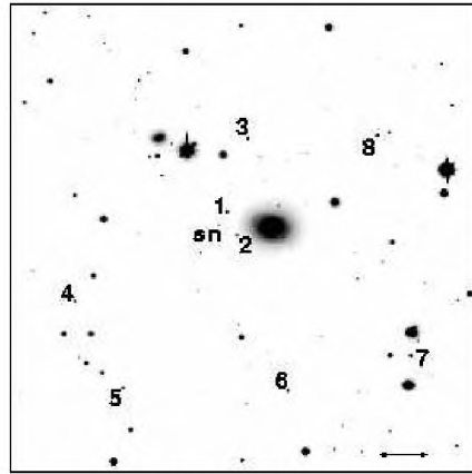
SN 1998de
