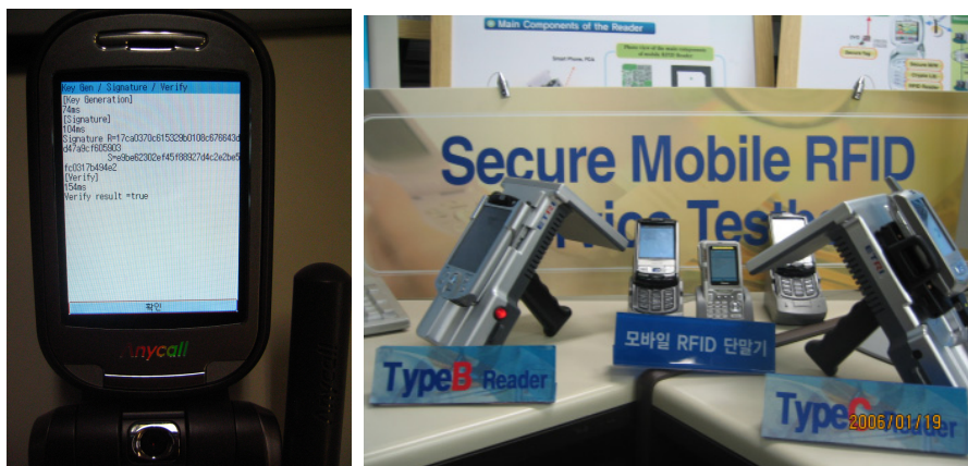
Fig. 7. UHF 900Mhz Mobile RFID Phone Reader
