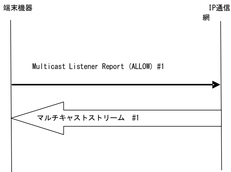
図2-2 マルチキャスト受信開始シーケンス例
