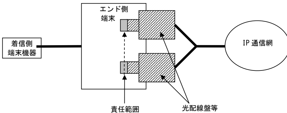
図 12-14 GigabitEthernet/10 GigabitEthernetタイプにおける施工・保守上の責任範囲分界点
