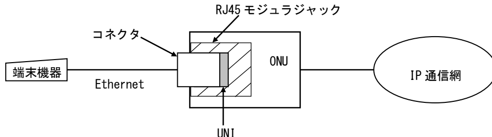
図 1-3 フレッツ 光クロスのインタフェース規定点
