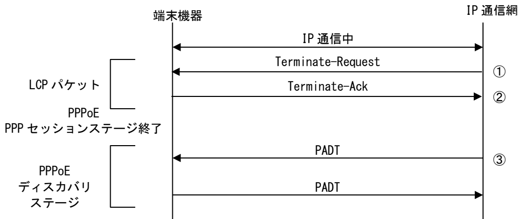
図 10-6 強制切断シーケンス (例)
