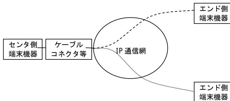
図 19-1 フレッツ・キャストの基本構成
