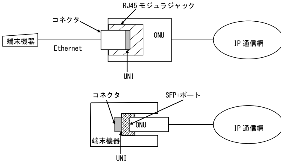
図 4-3 フレッツ 光ネクストのインターフェース規定点
