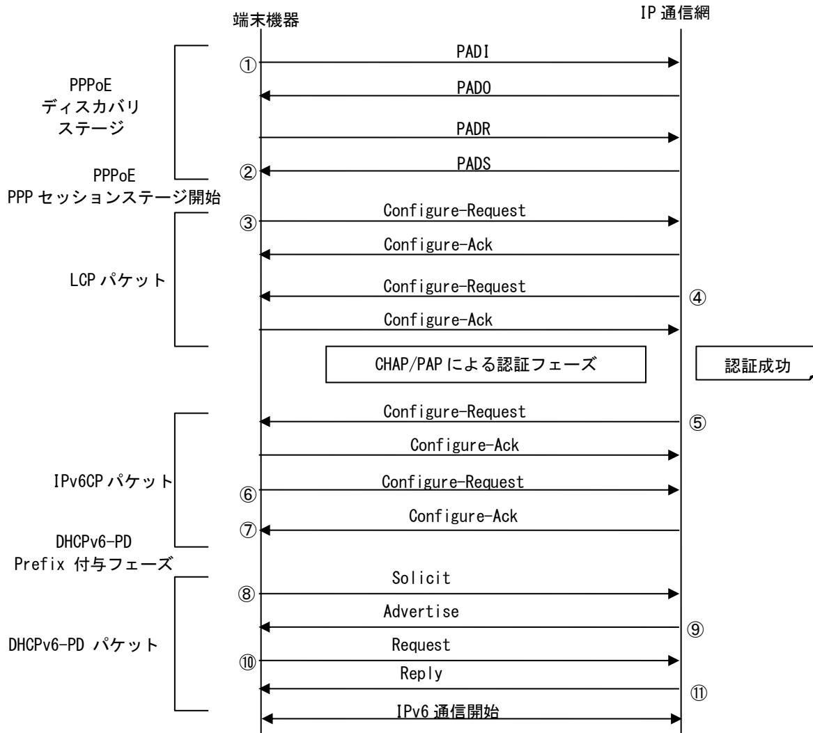
図 6-3 接続シーケンス (例)
