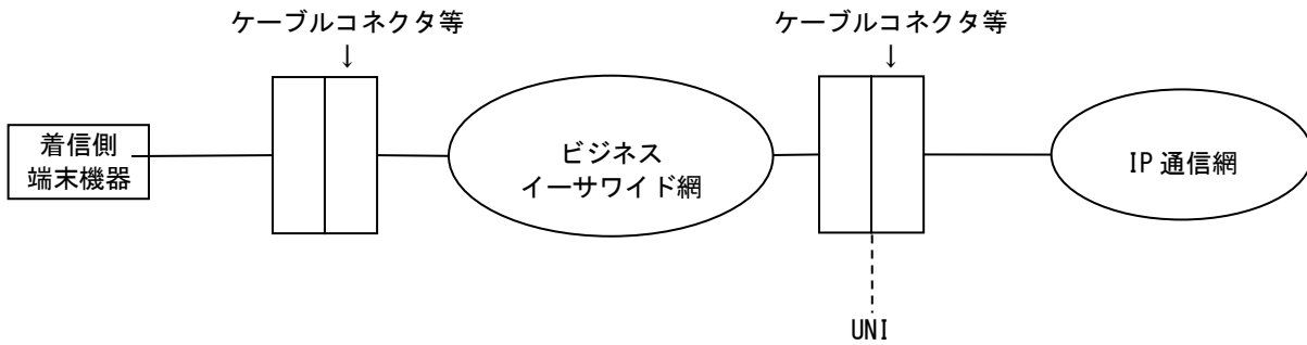
図 17-8 ビジネスイーサワイド接続タイプのインターフェース規定点
