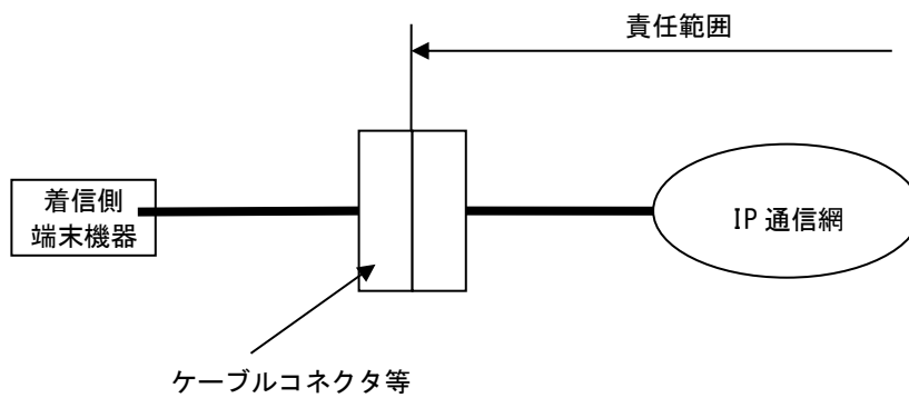
図 17-14 局内接続タイプの施工・保守上の責任範囲
