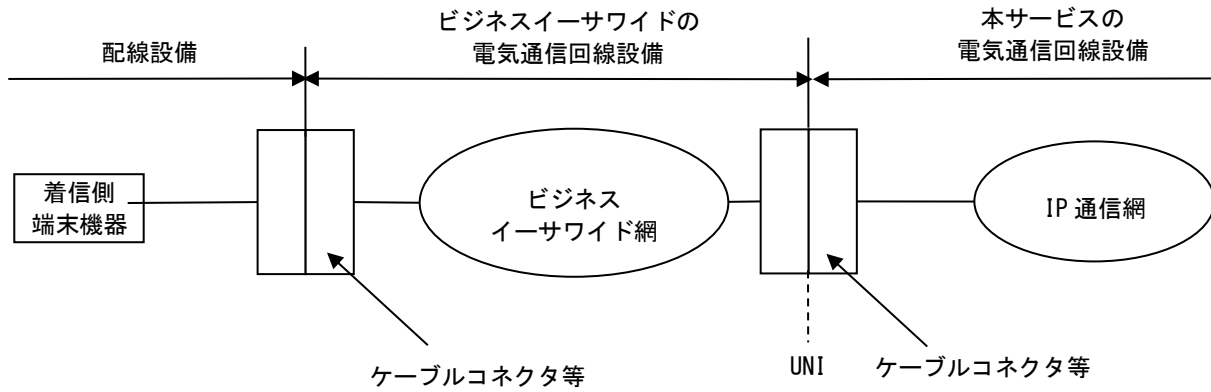
図 17-13 ビジネスイーサワイド接続タイプの分界点
