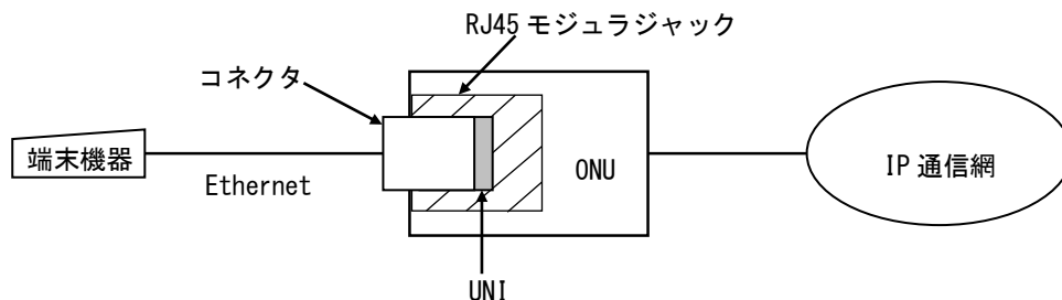
図 8-3 インタフェース規定点
