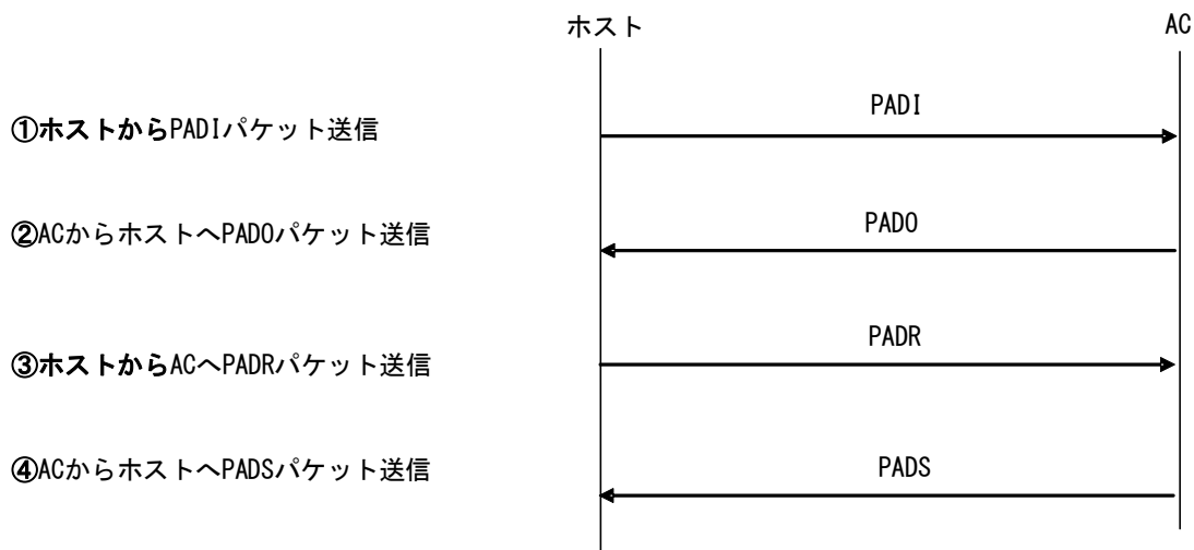
図 10-1 PPPoEセッション確立手順
