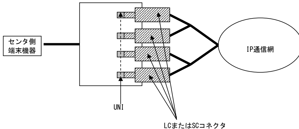
図 23-4 本サービスのインターフェース規定点
