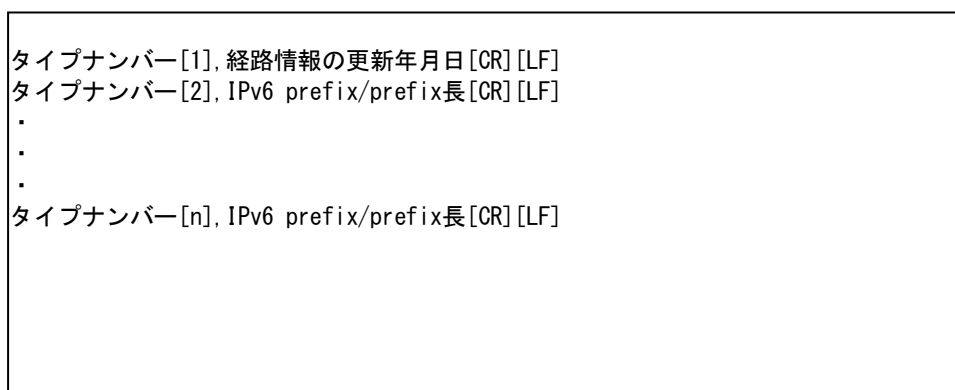
図 5-9 メッセージボディのフォーマット
