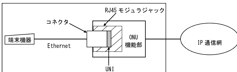
図 4-1 インタフェース規定点
