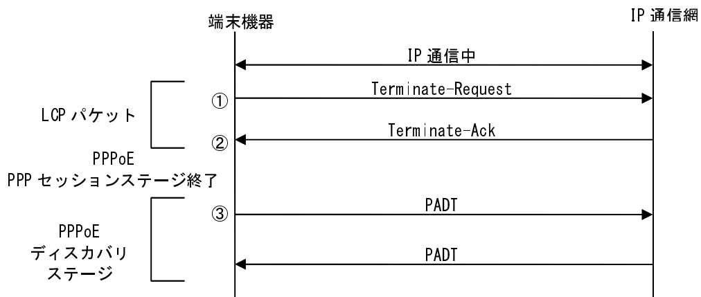
図 3-4 切断シーケンス (例)
