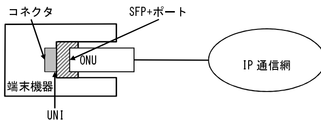
図 1-3 フレッツ 光ネクストのインタフェース規定点
