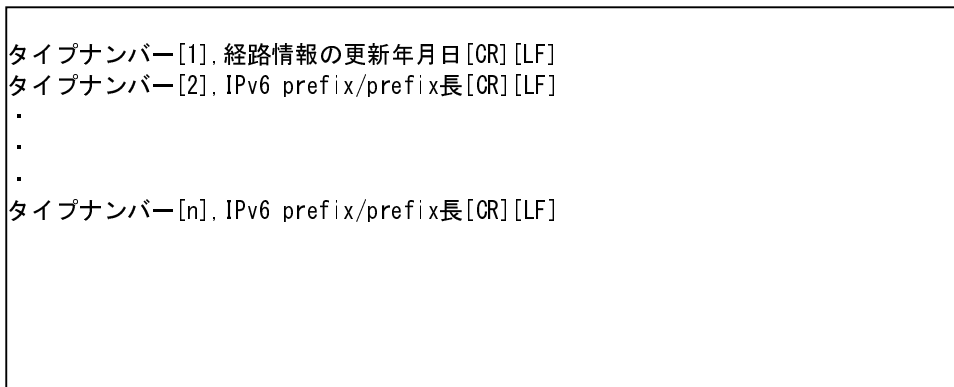
図 2-9 メッセージボディのフォーマット
