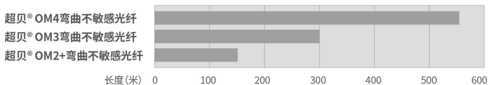
10 Gb/s 链路长度 (850nm)
