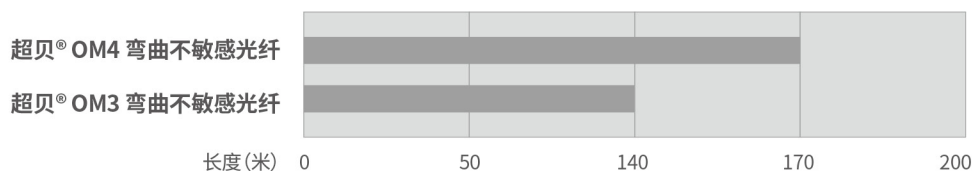
40 & 100 Gb/s 链路长度 (850nm)
