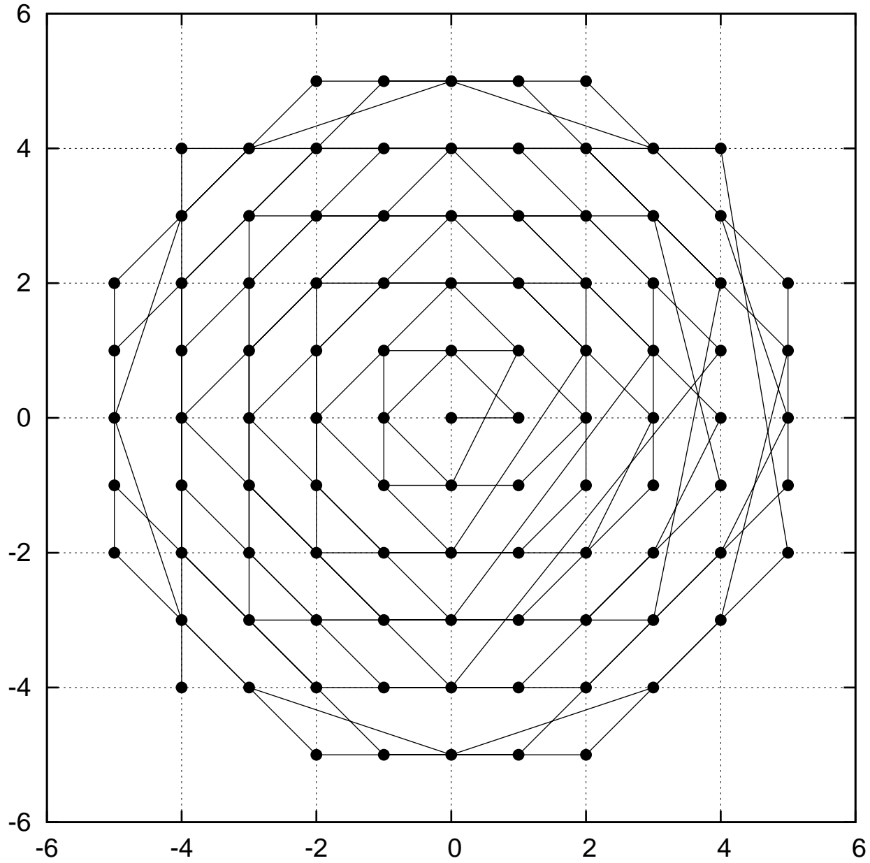
A305576 vs A305575
