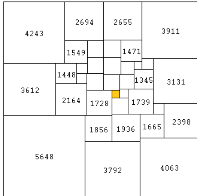
A349209(36) = 519
