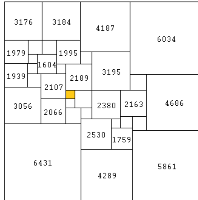
A349209(37) = 716
