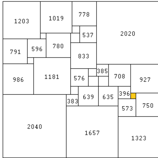
A349209(33) = 177
