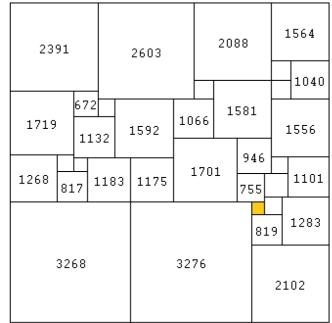
A349209(35) = 355
