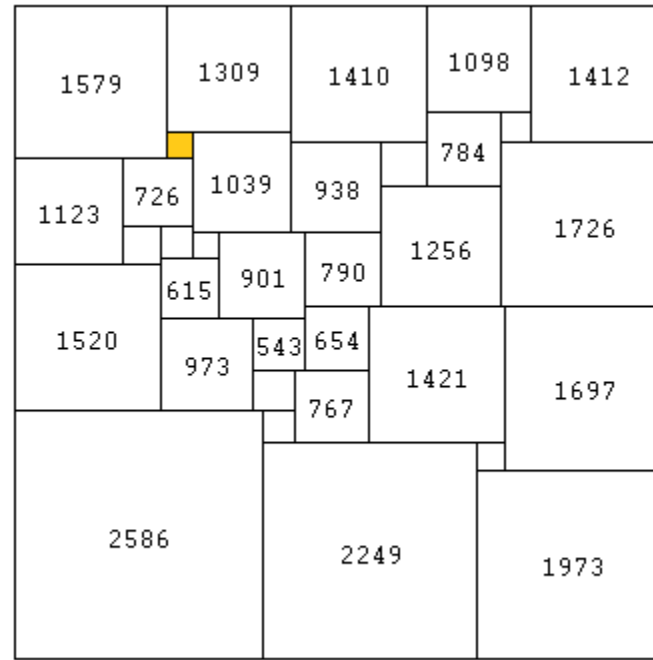
A349209(34) = 270
