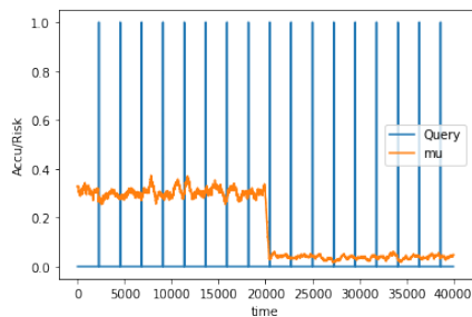
(d) PQ at \alpha=64 .
