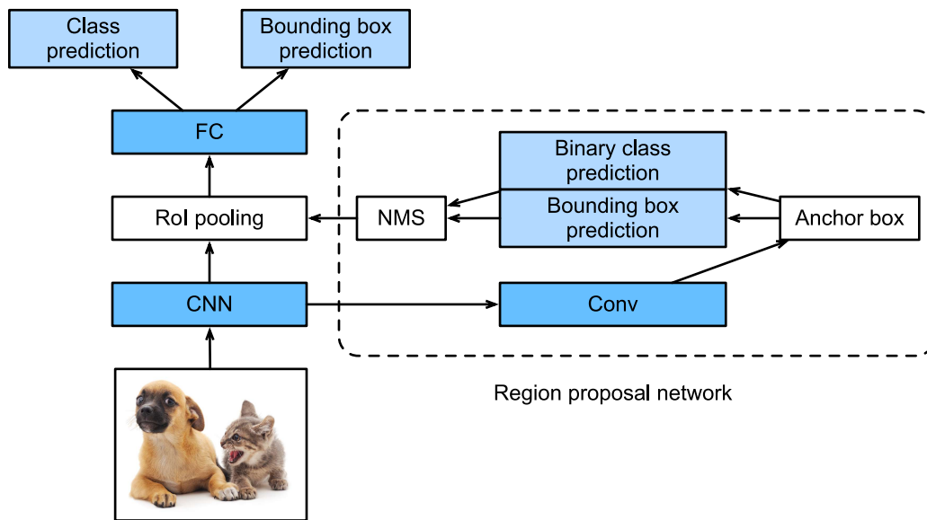
Fig. 13.8.4: Modelo R-CNN mais rápido.
