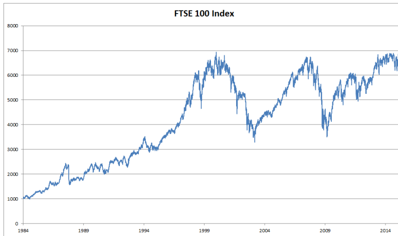
Fig. 8.1.1: Índice FTSE 100 ao longo de cerca de 30 anos.
