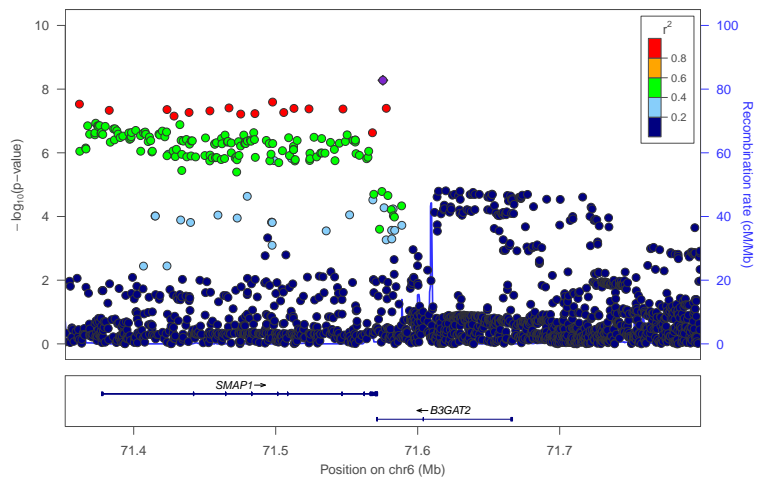
locus 220 rs9342993
