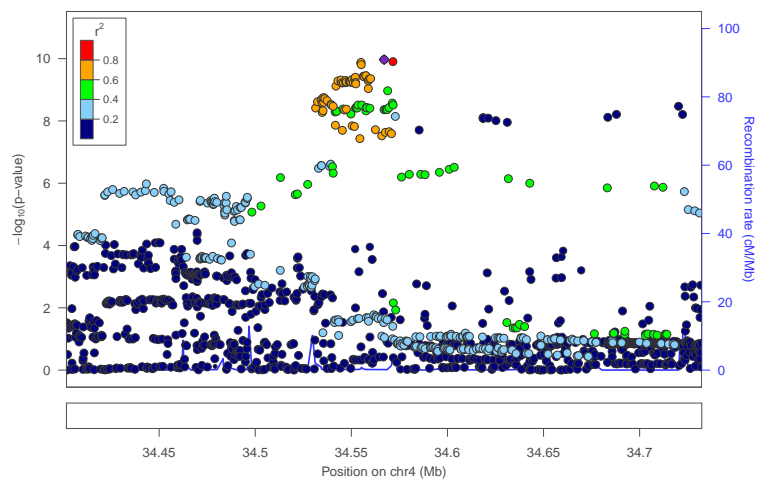
locus 145 rs10517119
