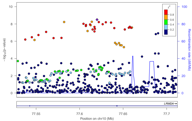
locus 346 rs188189626
