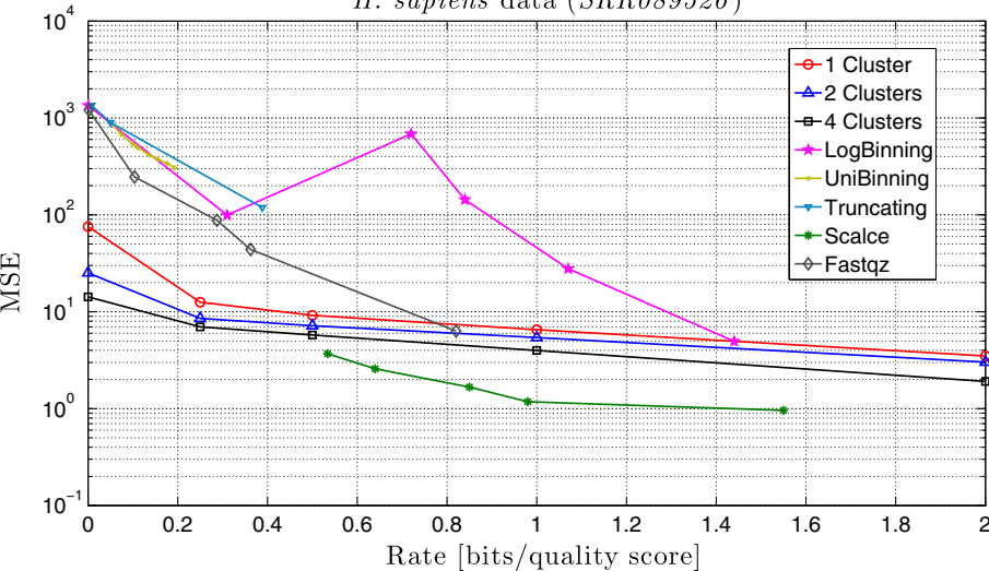
H. sapiens data (SRR089526)
