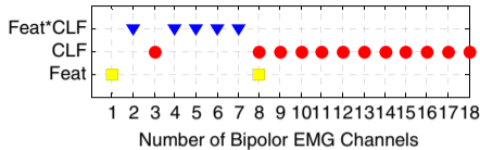
(b) MCCSP-Bipolar
