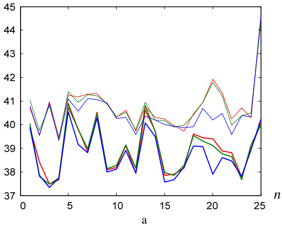
PSNR - HVS - M_k(n) , dB
