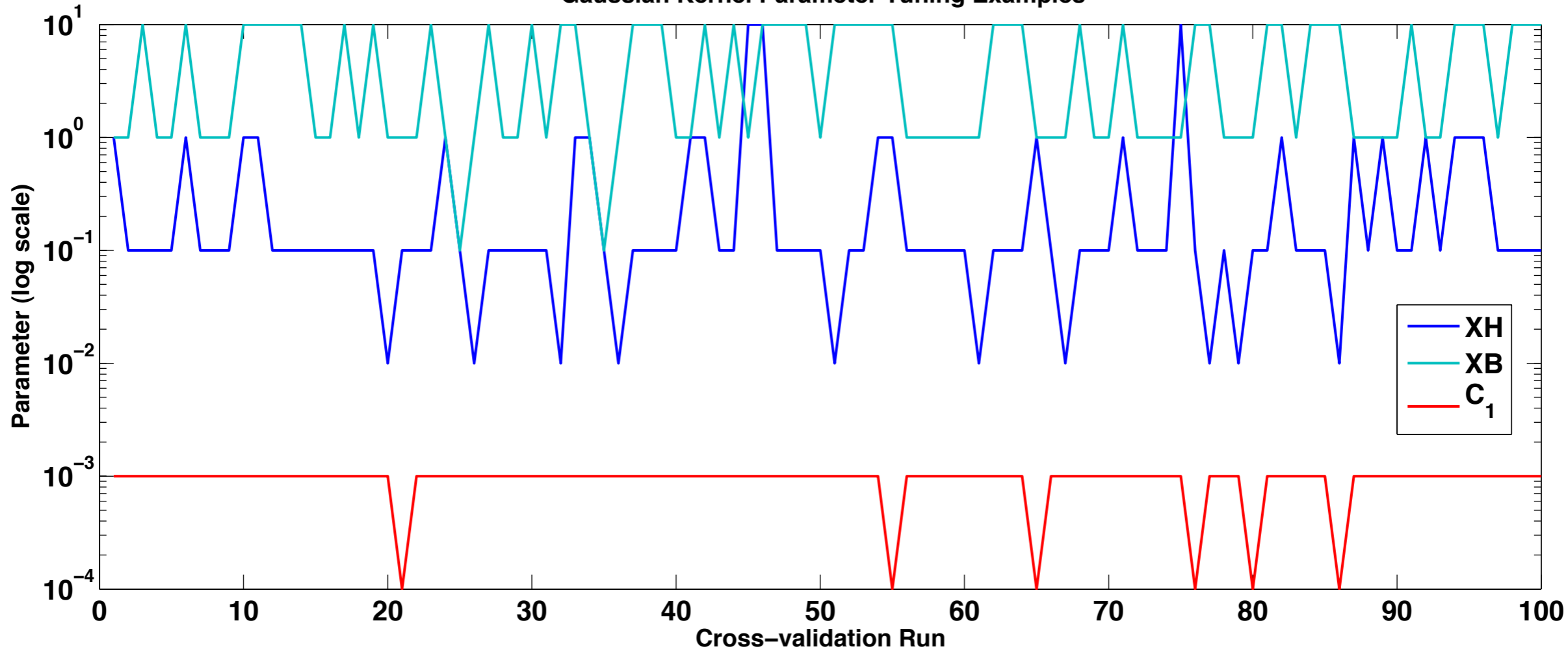
Gaussian Kernel Parameter Tuning Examples
