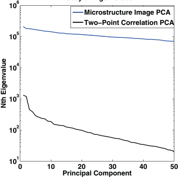
Decay of Eigenvalues
