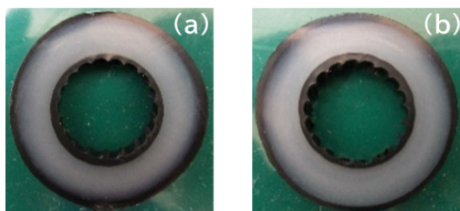
写真3 非架橋絶縁電力ケーブルの断面 (a) 短絡試験前、(b) 試験後
