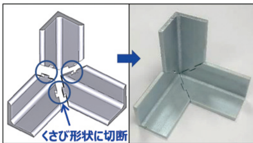
図3 はめ込み方式の切断事例
