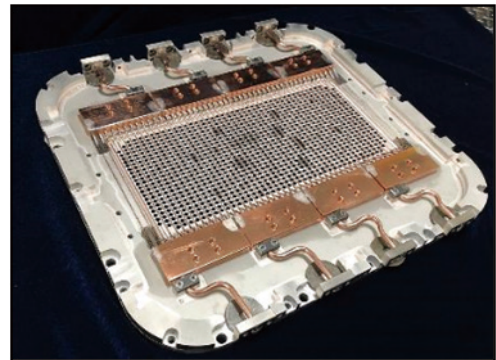
写真8 イオン源電極部品
