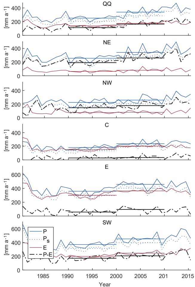
(b) MERRA-2
