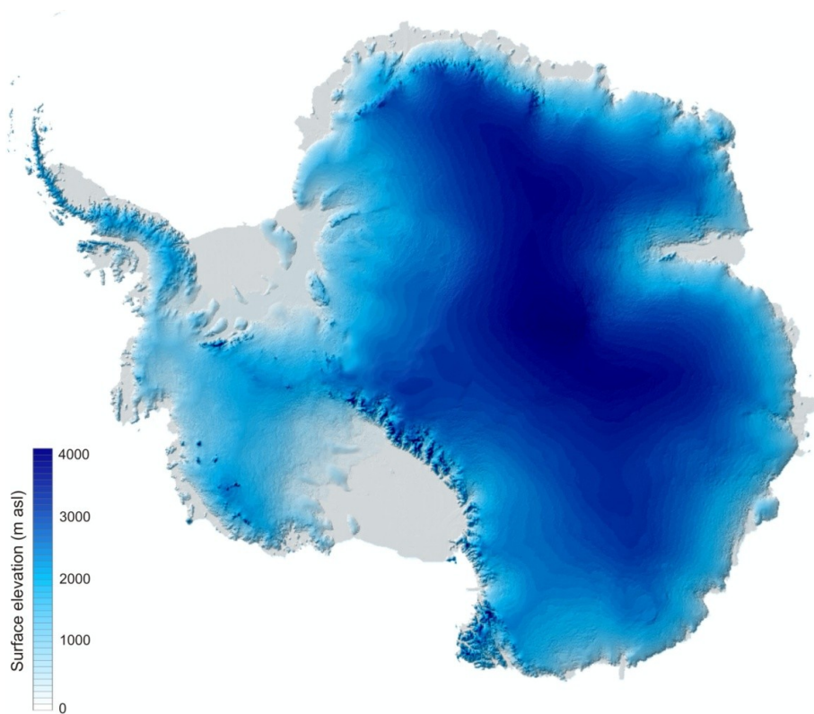
Fig. 7. Bedmap2 surface grid.
