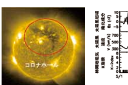
図3 SOHO衛星(ESA&NASA)の極端紫外線カメラで観測されたコロナホール(暗い部分)
