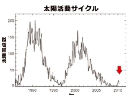
図1 太陽活動の指標となる太陽黒点数の月平均値の年々変化(データはSIDC、ベルギー王立天文台より)
