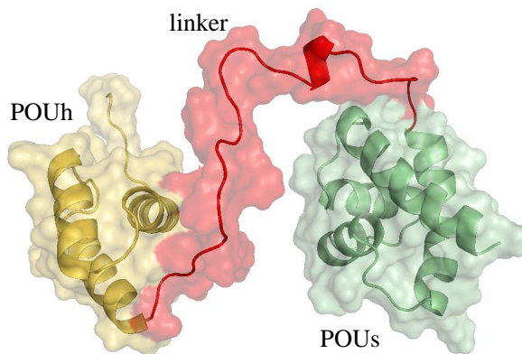
Fig. 5. Structure of N-Oct-3 POU domain.
