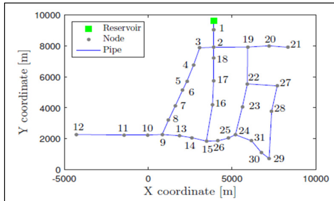
Fig. 4: Hanoi WDN.
