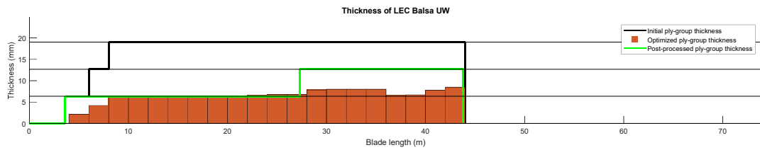
(d) Leading edge core balsa upwind.
