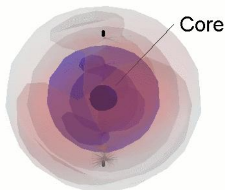
A.I.Dubinyansky @ P.A.Churlyayev. Внутренняя структура нейтрона.
