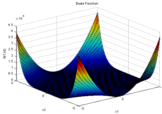
Fig. 3. Beale function
