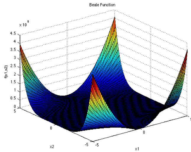
Fig. 2. Beale Function
