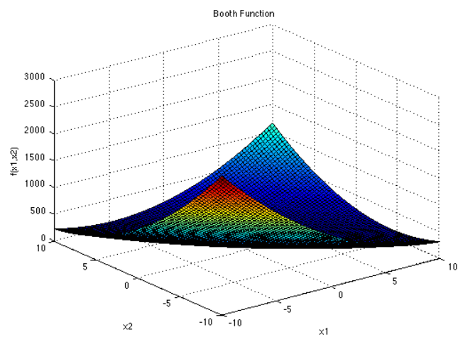
Fig. 4. Booth Function
