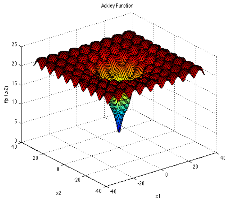
Fig. 1. Ackley Function
