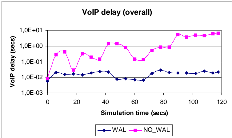
(a) VoIP delay
