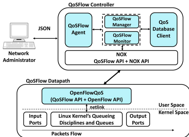
Fig. 18. QoSFlow modules [134].
