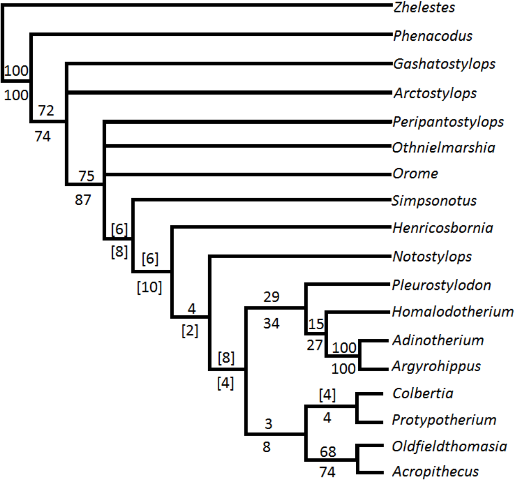
SOM 1. Consensus tree
