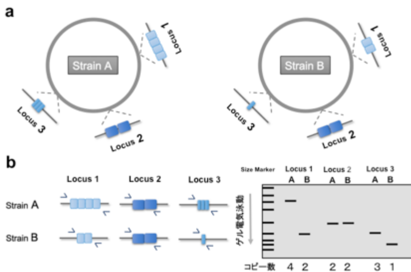
図1. VNTR法の概容 a: 検査対象のVNTR領域、b: PCRによるVNTR領域の増幅と電気泳動によるPCR産物の分子量(bp)の測定、及び反復配列の反復数(コピー数)の算出
