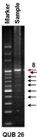
図. Stutter peak の例。黒矢印の部分に stutter peaks が検出されており、反復数を逆算出来ることが分かる。QUB 26 領域の反復数 8 と判定。
