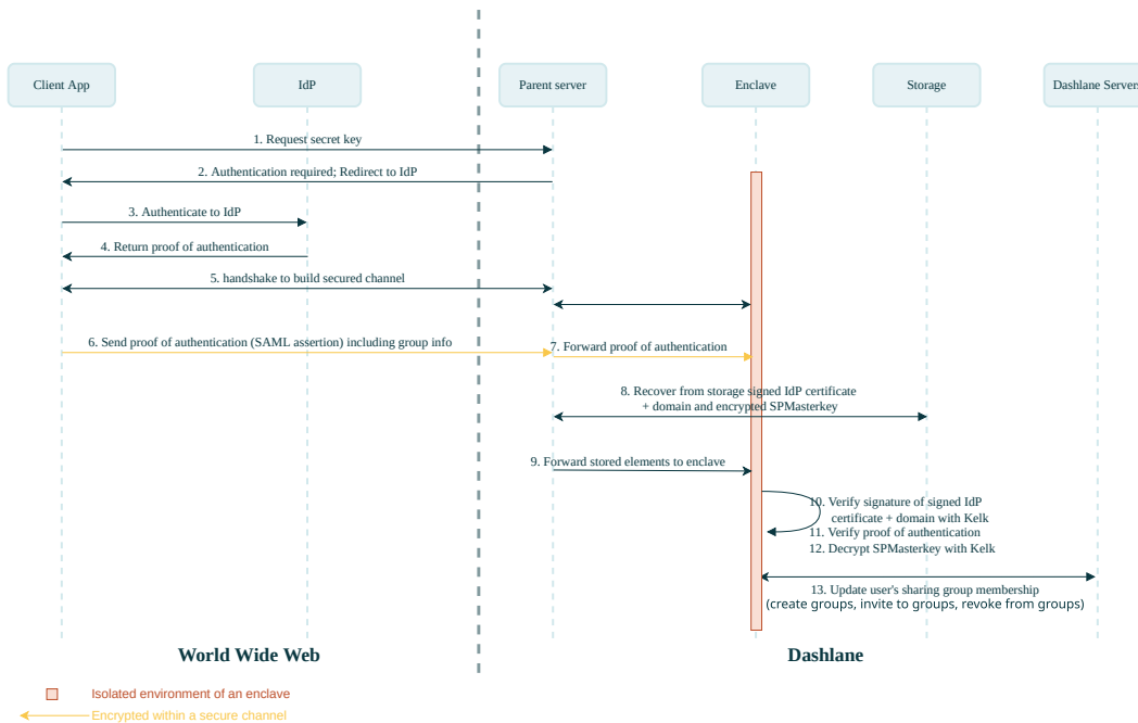
Fig. 12 : Provisionnement "confidentiel" de groupes de Dashlane
