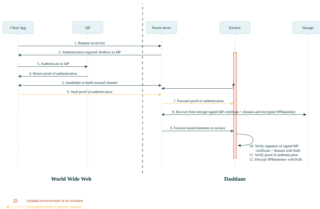
Fig. 9 : Confidential SSO de Dashlane - Flux de connexion de l'utilisateur
