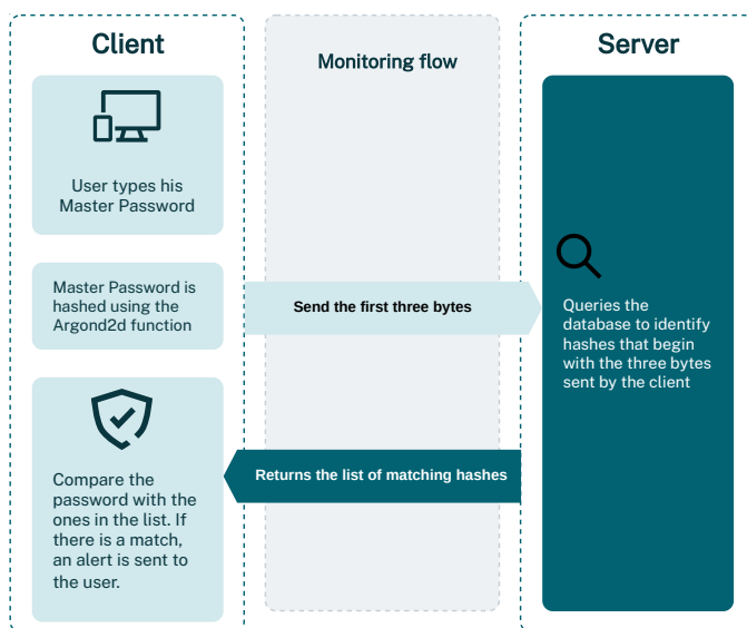
Fig. 4 : Surveillance du dark Web pour le flux de mots de passe Maître
