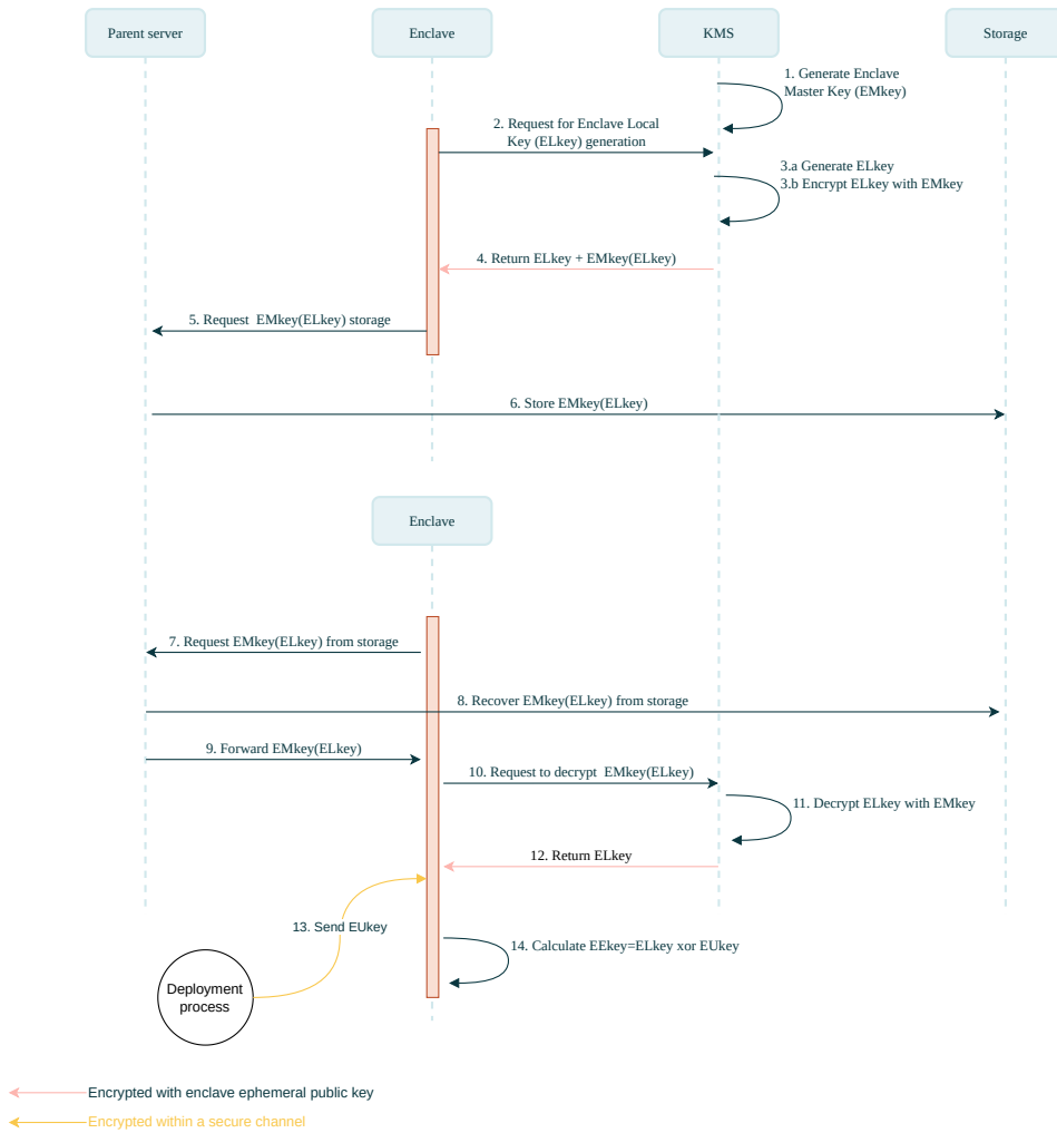
Fig. 7 : Initialisation de la Dashlane Confidential SSO
