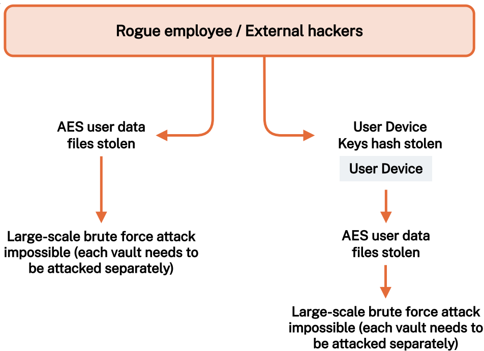
Fig. 15 : Scénarios d'attaque avec l'architecture de sécurité de Dashlane
