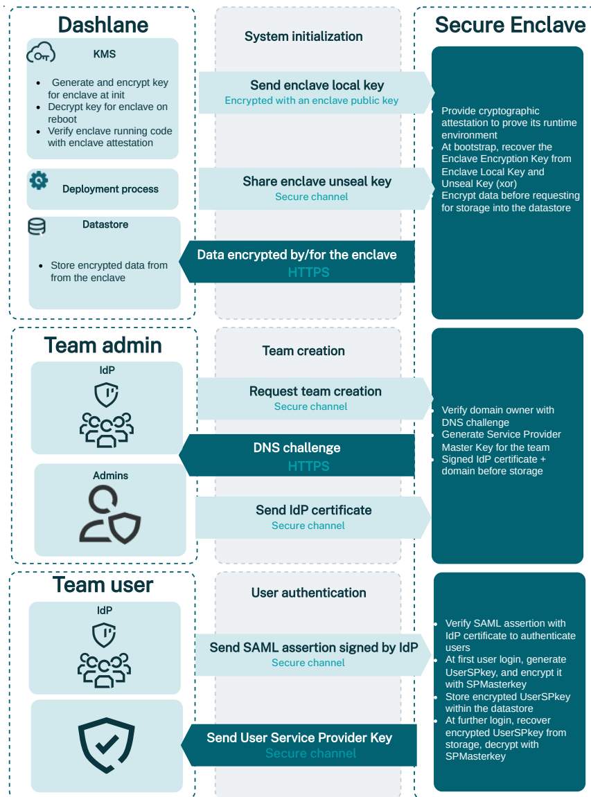
Fig. 6 : Flux de travail SSO hébergés par Dashlane
