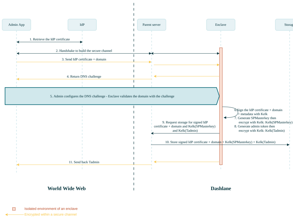
Fig. 8 : Flux de création d'une équipe avec Dashlane Confidential SSO
