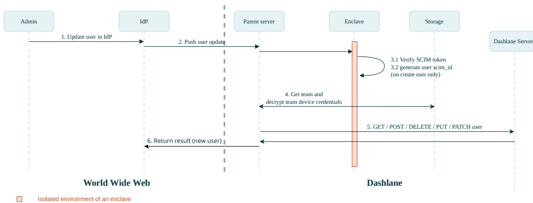
Fig. 11 : Provisionnement "confidentiel" d'utilisateurs de Dashlane
