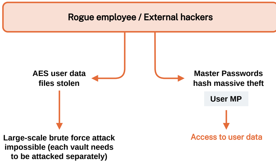
Fig. 14 : Scénarios d'attaque avec la plupart des architectures cloud
