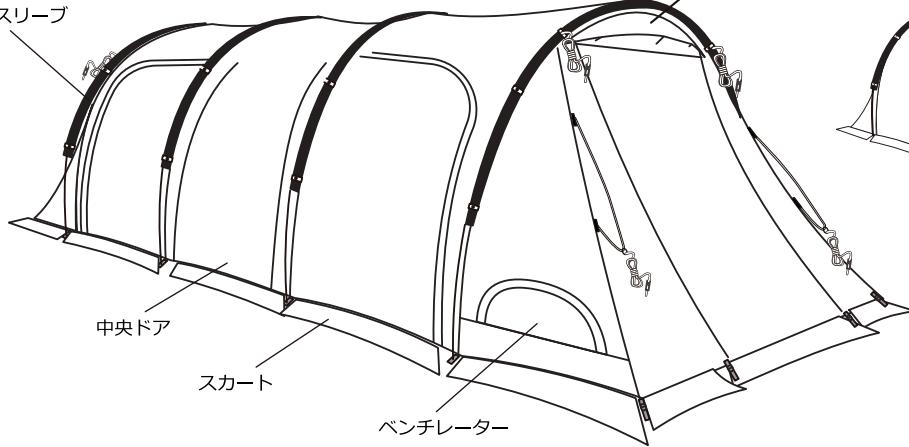
1 アウターテント
