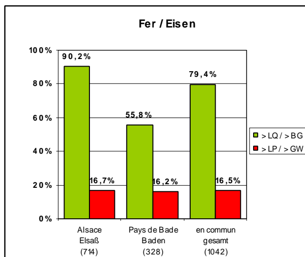
Fig. 3.3.34 : Pourcentage des concentrations en fer supérieures à la limite de quantification (LQ) et supérieures à la limite de potabilité (LP) (avec indication du nombre de points de mesure)
