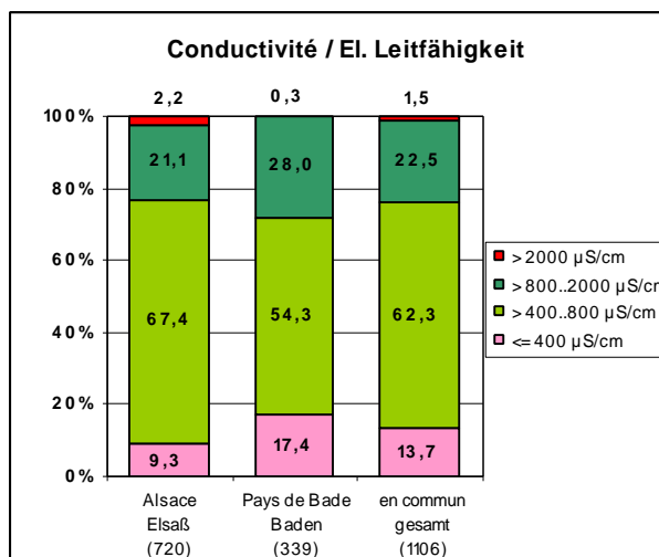
Fig. 3.2.4: Répartition des valeurs de la conductivité (avec indication du nombre de points de mesure)
