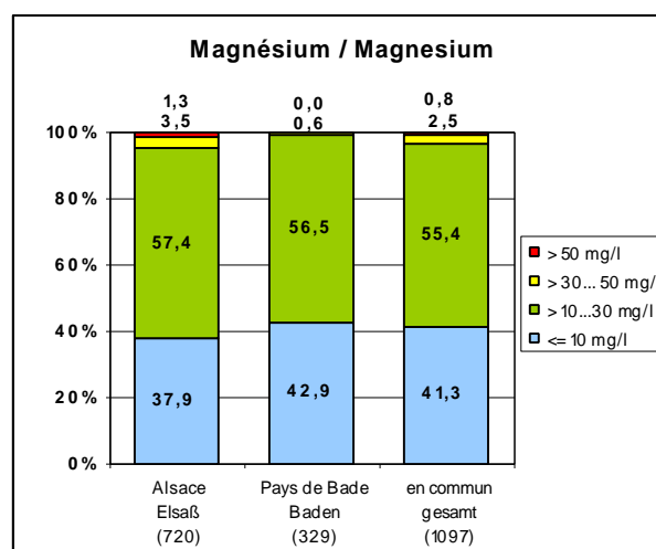
Fig. 3.2.16: Répartition des concentrations en magnésium (avec indication du nombre de points de mesure)
