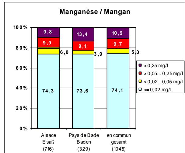
Fig. 3.2.37 : Répartition des concentrations en manganèse (avec indication du nombre de points de mesure)
