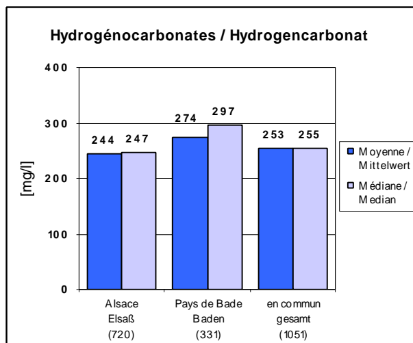
Fig. 3.2.11 : Moyennes et médianes de la répartition des concentrations en hydrogencarbonates (avec indication du nombre de points de mesure)
