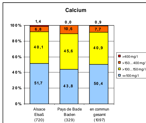
Fig. 3.2.14: Répartition des concentrations en calcium (avec indication du nombre de points de mesure)
