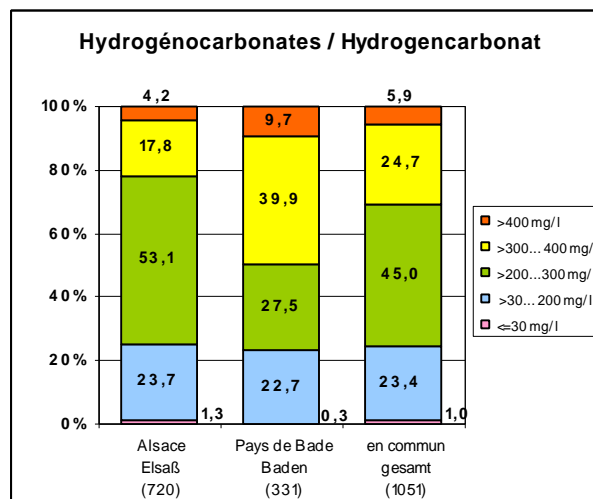
Fig. 3.2.12: Répartition des concentrations en hydrogencarbonates (avec indication du nombre de points de mesure)
