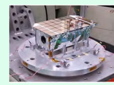
近赤外分光計 NIRS3
