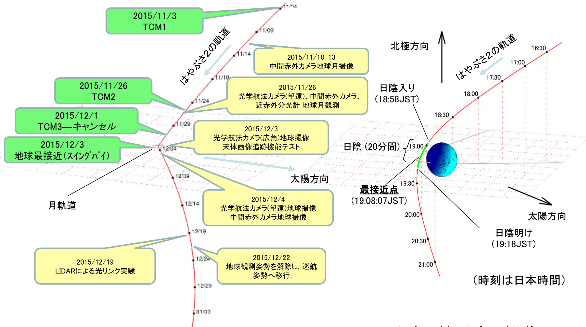
地球スイングバイの前後での主な運用
