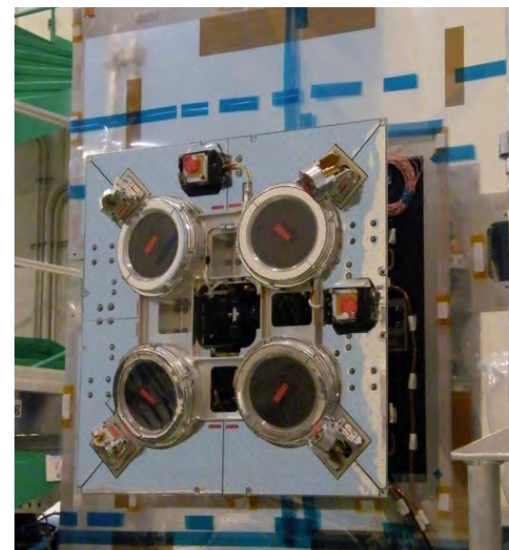
はやぶさ2イオンエンジン
