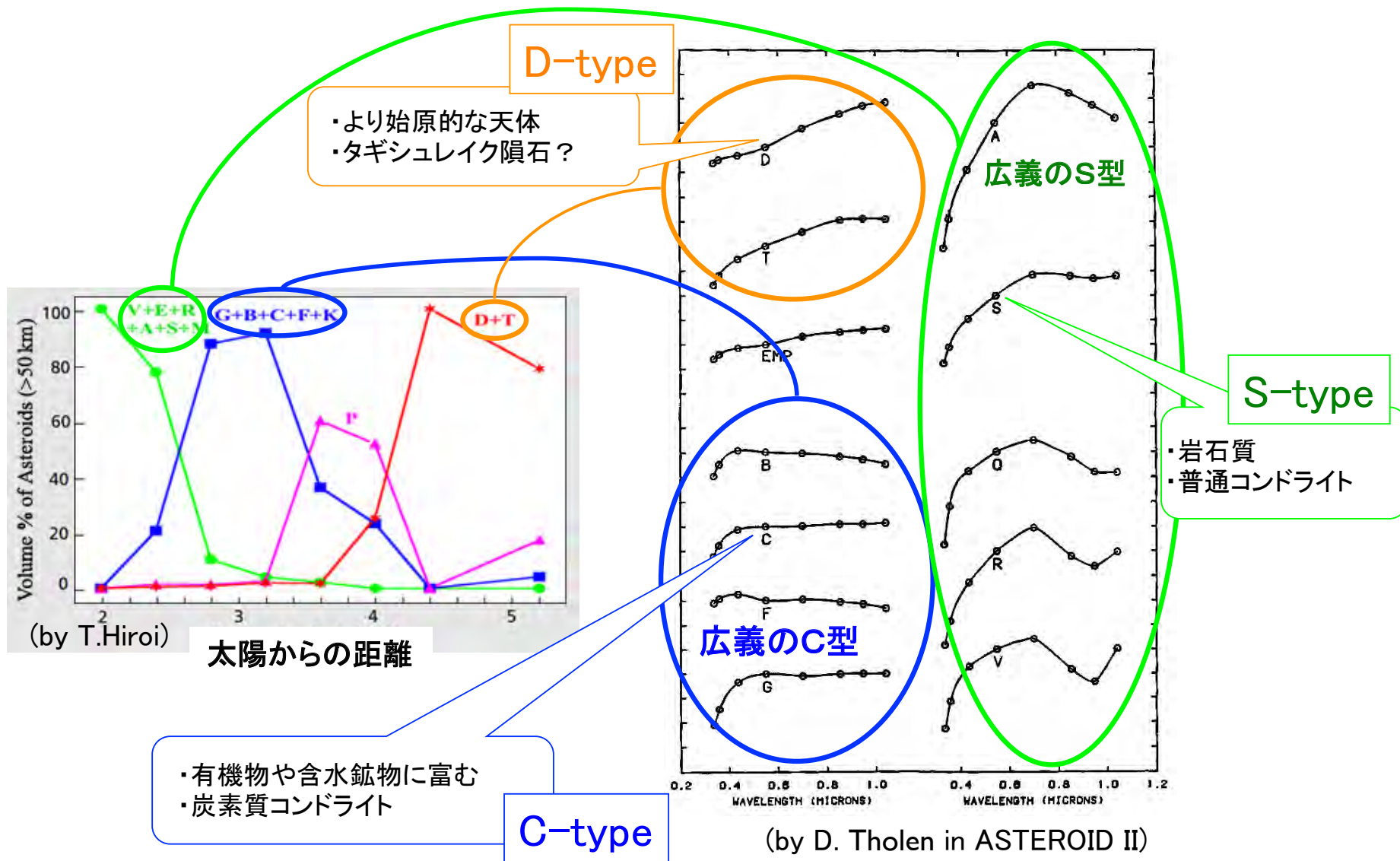
反射スペクトルによる小惑星の分類
