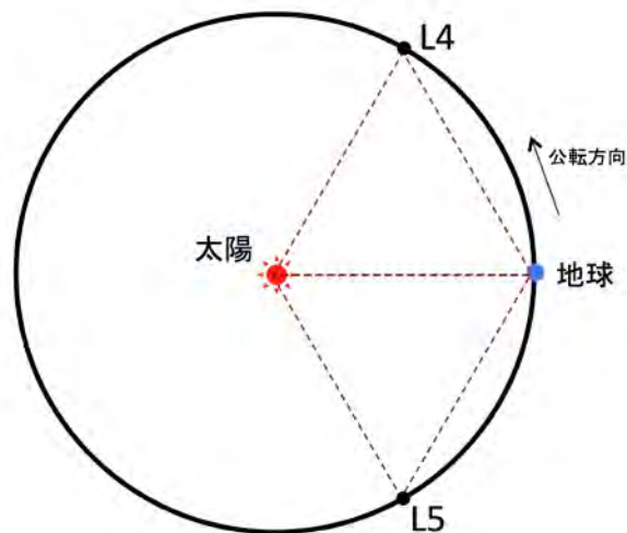
太陽-地球系のラグランジュ点L4、L5
