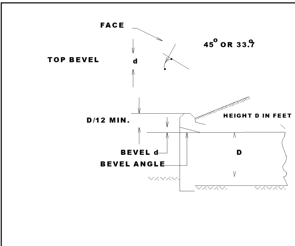
Inlet Top Edge Bevel (Chart 9)
