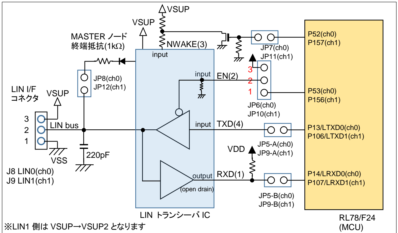
図 2-5 LIN インタフェースブロック図
