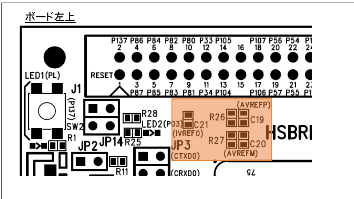
図 2-7 VREF 向け容量、抵抗ランドパターン
