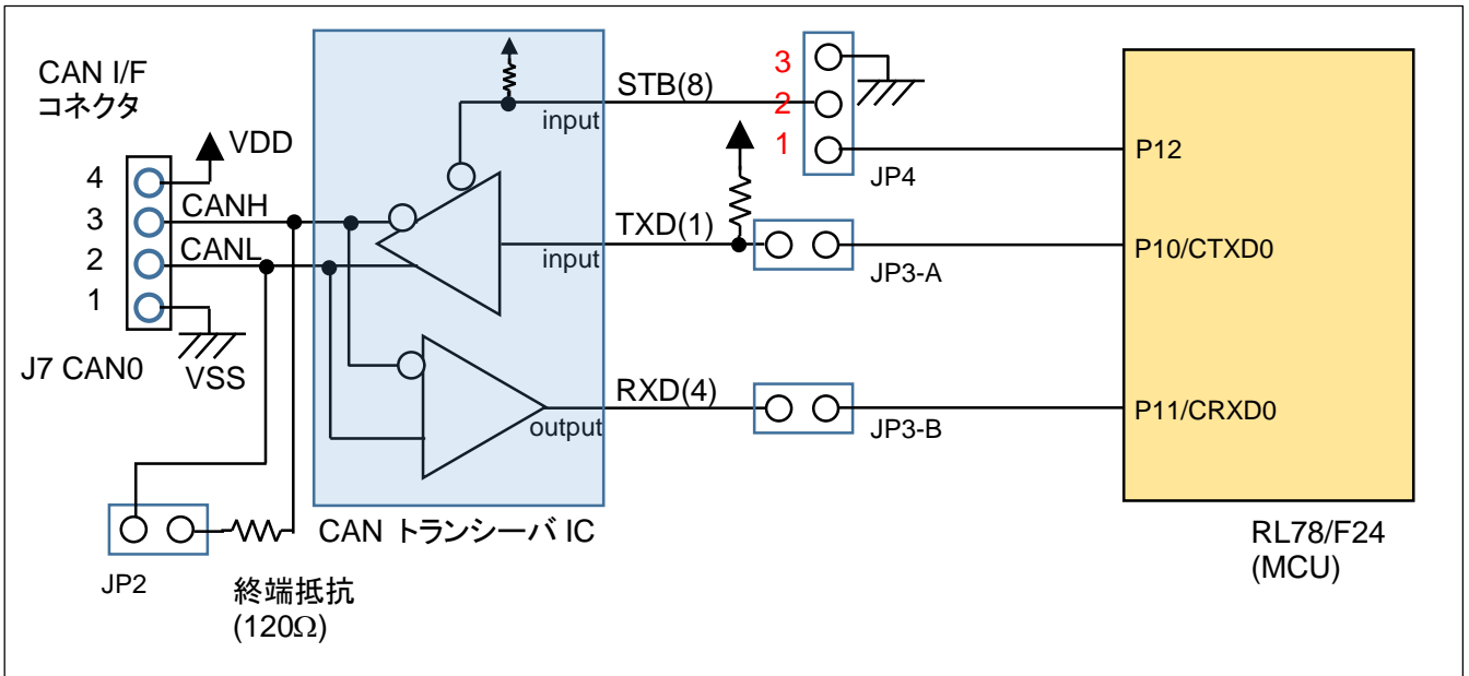
図 2-4 CAN インタフェースブロック図
