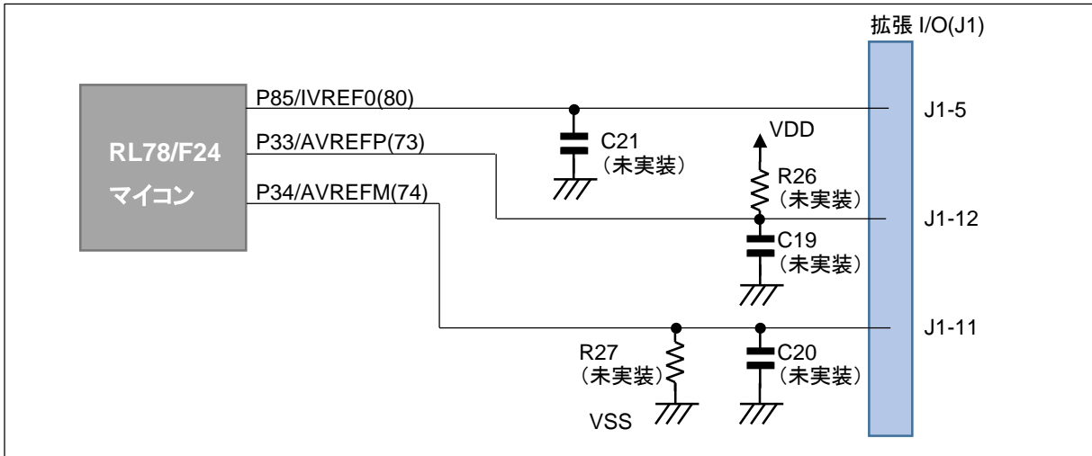
図 2-6 VREF 部回路
