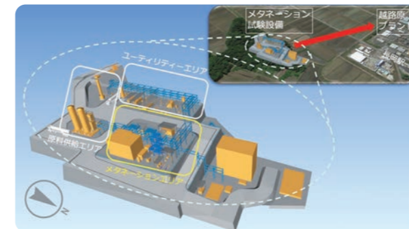
現在建設中の400Nm 3 /hプラントモデル図
